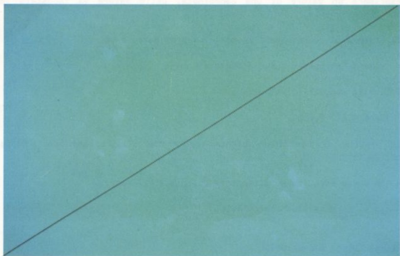
Figura 14-11 Istruzione LINE
